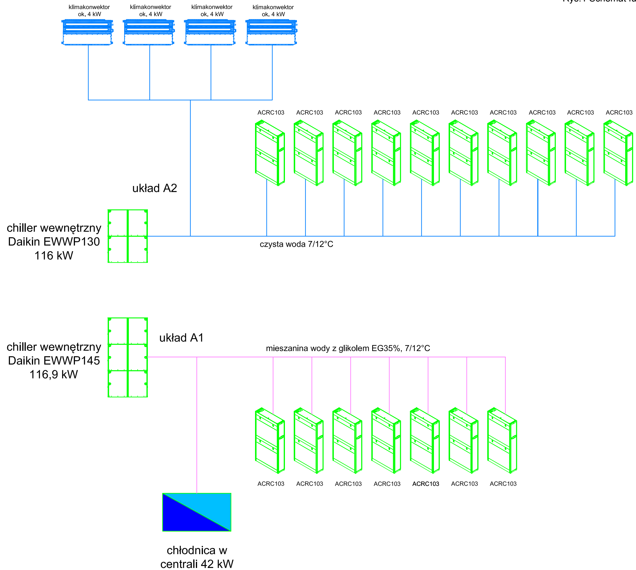
Rys.1 Schemat funkcjonalny - Stan istniejący
