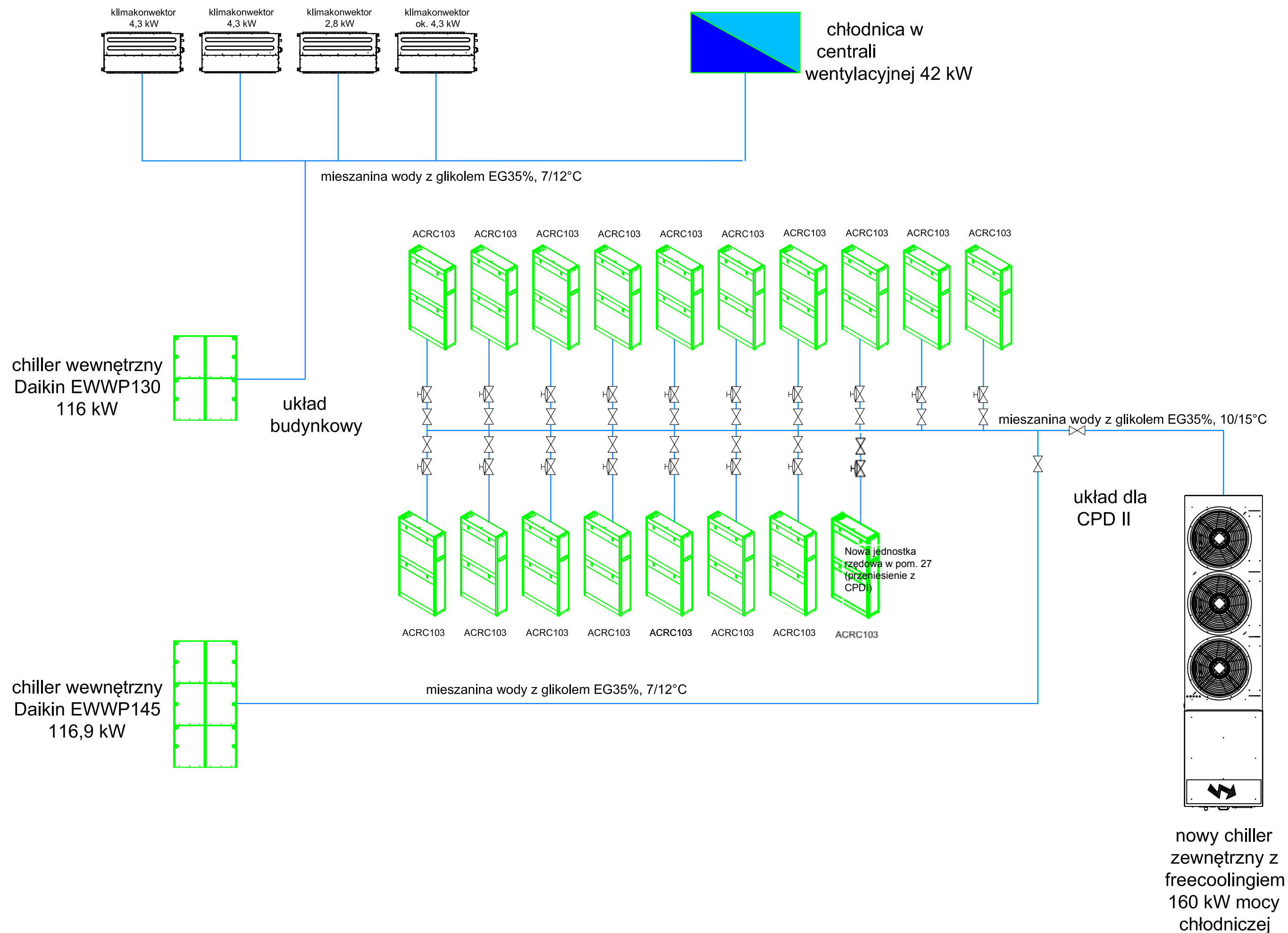
Rys. 2 Schemat funkcjonalny - Stan docelowy
