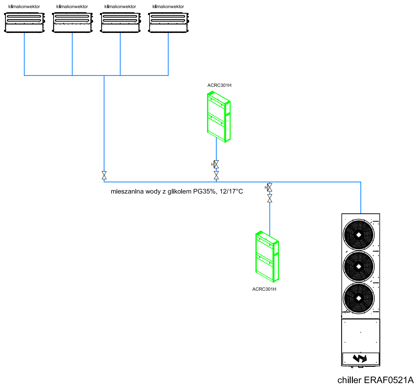
Rys.2: Schemat funkcjonalny -Stan docelowy
