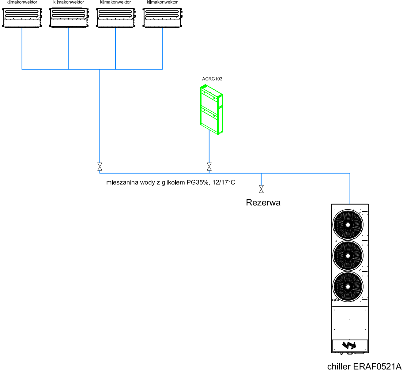
Rys.1: Schemat funkcjonalny - Stan istniejący
